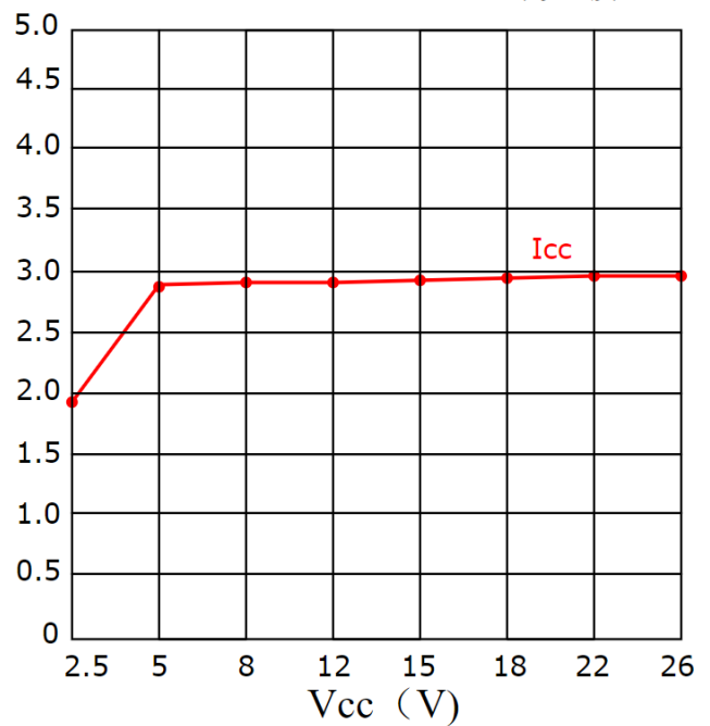
功耗电流mA 环境温度25°C
